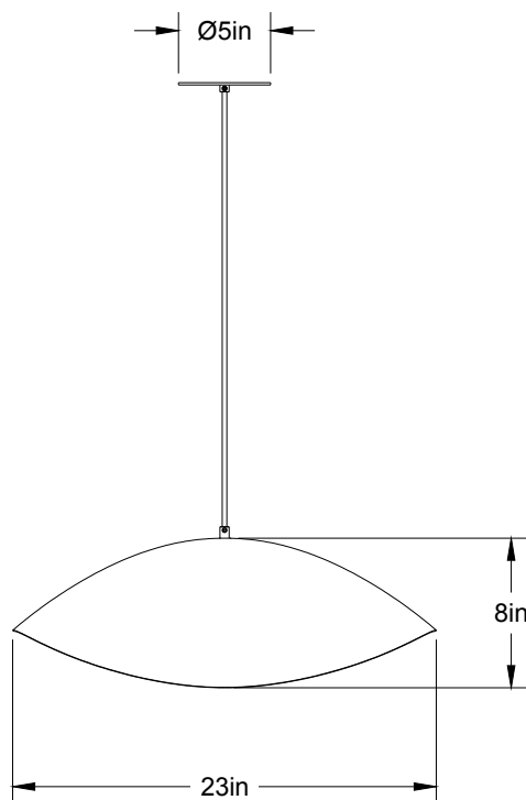
Avant/Front
