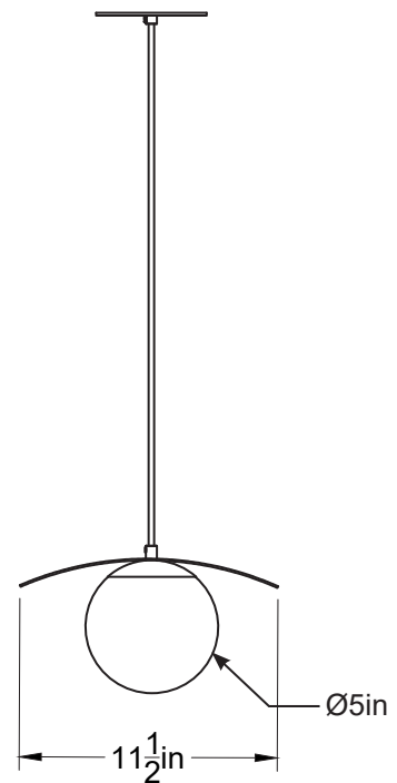
Côté/Side
