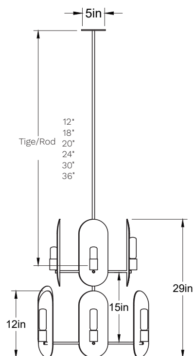
Avant/Front
