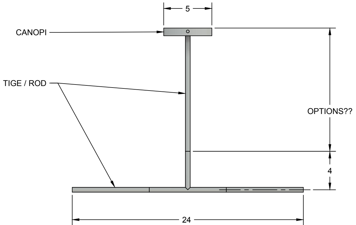
CÔTÉ / SIDE
