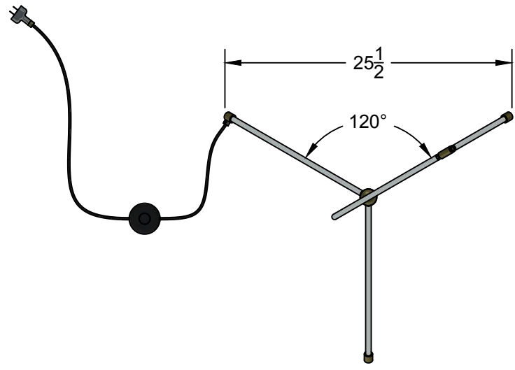
DESSUS / TOP
